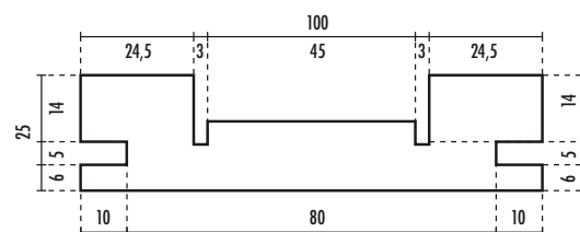
A montante telaio
