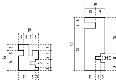
B montante battuta
