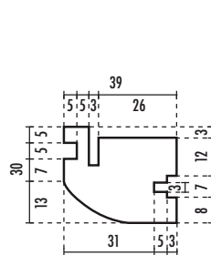
B montante telaio
