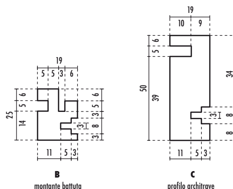
Bino's per cartongesso monoanta - mm. 100
